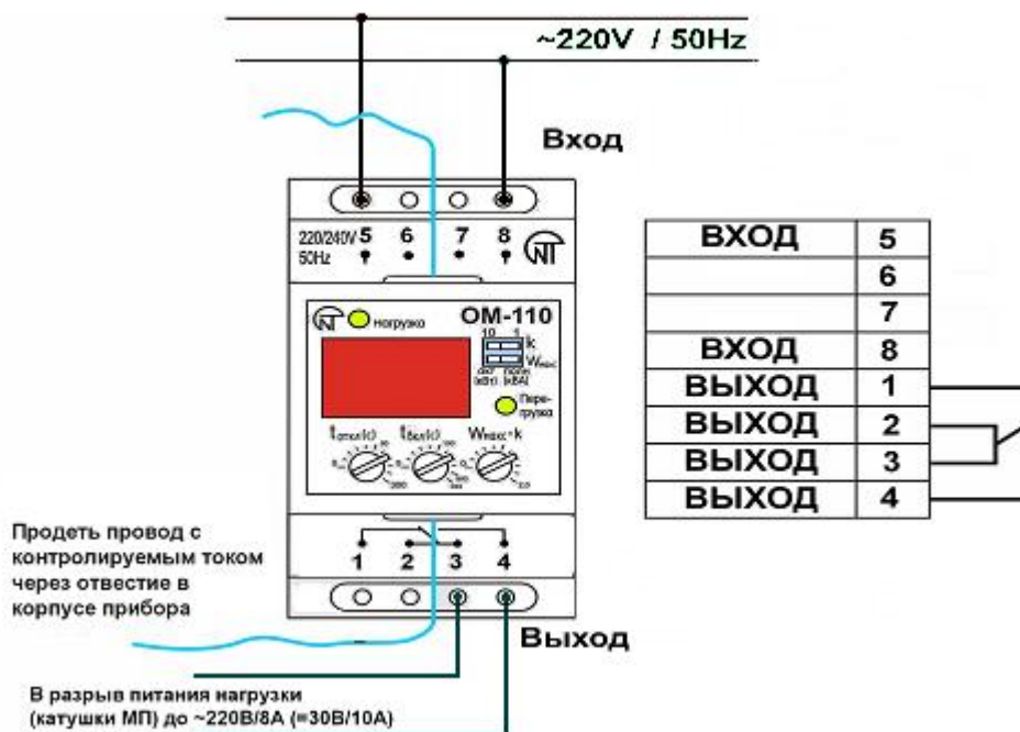
Рисунок 2 - Схема подключения ОМ-110
