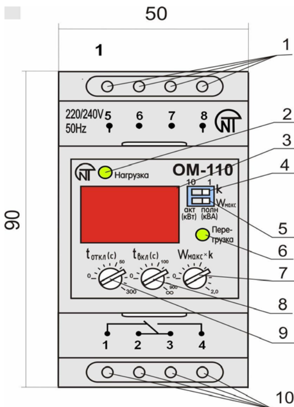
Рисунок 1 - Внешний вид ОМ-110
